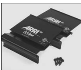
L4.79427UE Set of side panels (USA) ETL (to ser.no.8137) black Set Seitenbleche (USA) ETL (bis Ser.Nr.8137) schwarz
