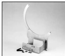
L4.81398.E from ser. no. 774 Spindle/Spindel: 16 mm Lamp carriage Fokusschlitten
