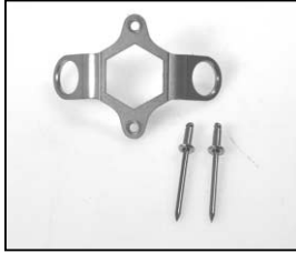
L4.70854.E Strain relief fixing for PG11 strain relief (Par to serial No. 714, Lite to serial No. 367, lamp housing to serial No. 215) Sicherungsöse für Zugentlastung PG11 (Par bis Serien Nr. 714, Lite bis Ser.Nr. 367, Lampengehäuse bis Ser.Nr. 215)
