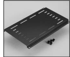
L4.83216.E Bottom panel Bodenblech
