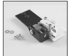
L4.73417SE Safety switch H.T. complete Endschalter H.T. komplett
