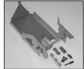
L4.81088.E Reflector holder for rear loader versions Reflektorhalter für Hecklader Version
