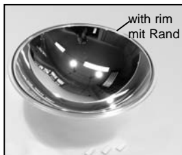
L4.80112.E New glass reflector from ser. no. 479 (does not fit into reflectorholder to ser. no. 478 - in this case please order L4.80769.E) Glasreflektor neu ab Ser. Nr. 479 (passt nicht in Reflektorhalter bis Ser. Nr. 478 - in diesem Falle bitte L4.80769.E bestellen)
