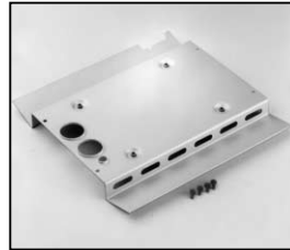
L4.74018.E Intermediate panel Zwischenblech
