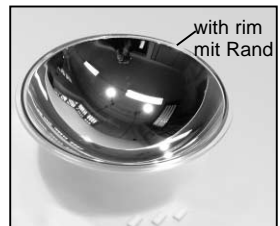
L4.80112.E New glass reflector from ser. no. 364 (does not fit into reflector holder to ser. no. 363 - in this case please order L4.80769.E) Neuer Glasreflektor ab Ser. Nr. 364 (passt nicht in Reflektorhalter bis Ser. Nr. 363 - in diesem Falle bitte L4.80769.E bestellen)
