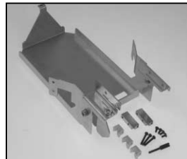
L4.81088.E Reflector holder for rear loader versions Reflektorhalter für Hecklader Version
