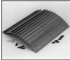
L4.83274.E Side extrusion compl.left "door-catch-side" Rippenblech kpl.links "Verschlußseite"
