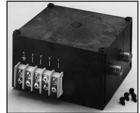
L4.83258.E Ignitor Zündgerät
