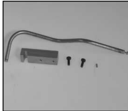
L4.81129.E Safety switch activator, rear for rear loader versions Drahtauslöser, hinten für Hinterlader Version
